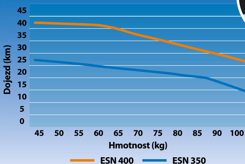
Dojezd (km) v závislosti na hmotnosti (kg)
