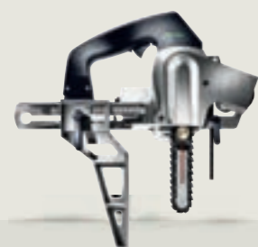
Řetězová dlabačka CM 150
